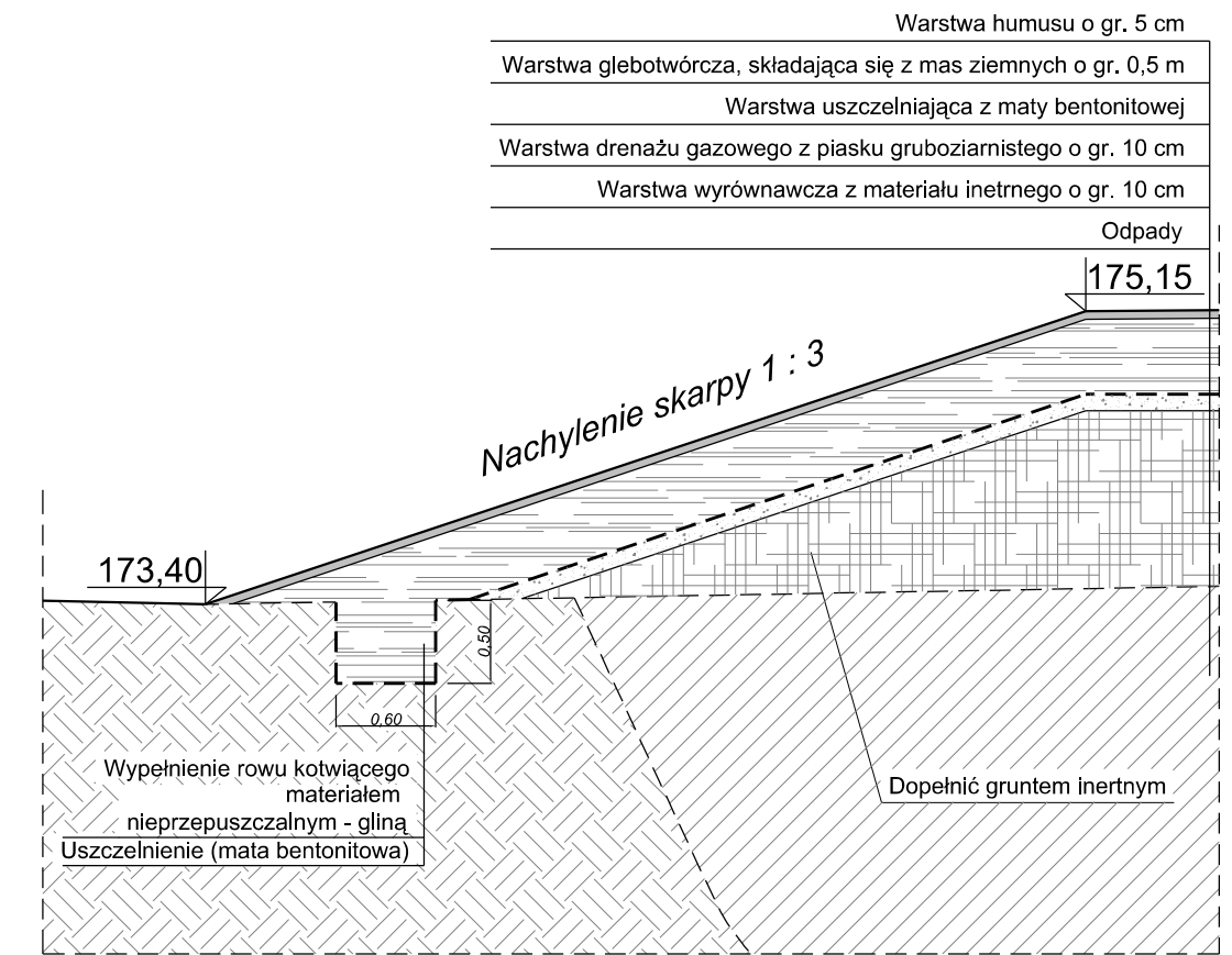
SZCZEGÓŁ "C" 1 : 50
