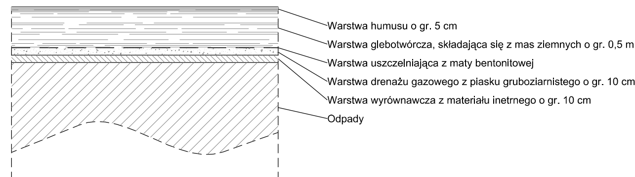
PRZEKRÓJ PRZEZ OKRYWĘ REKULTYWACYJNĄ 1 : 50
