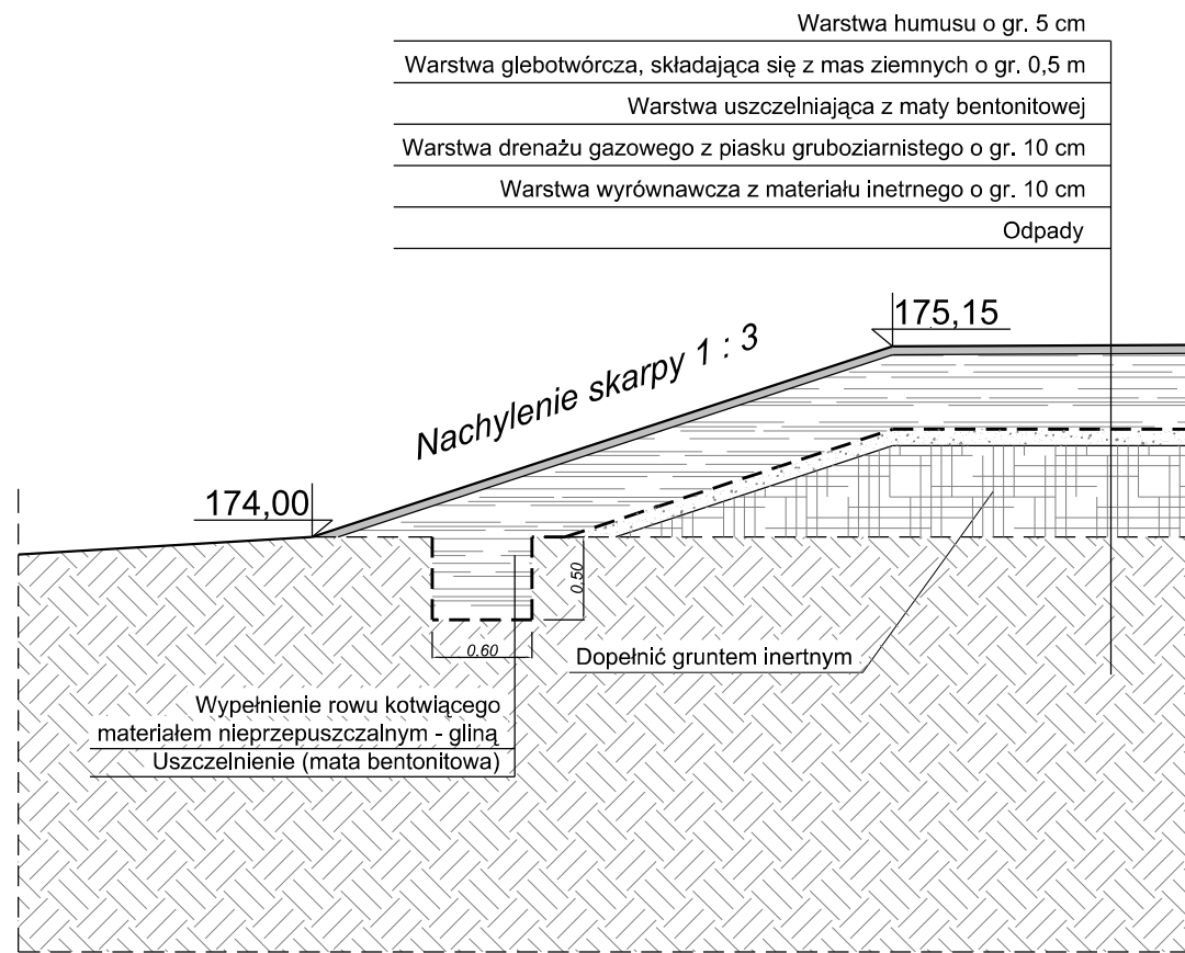
SZCZEGÓŁ "A" 1 : 50
