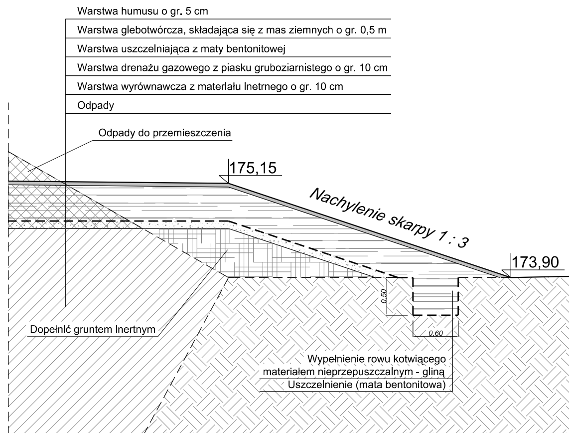
SZCZEGÓŁ "D" 1 : 50
