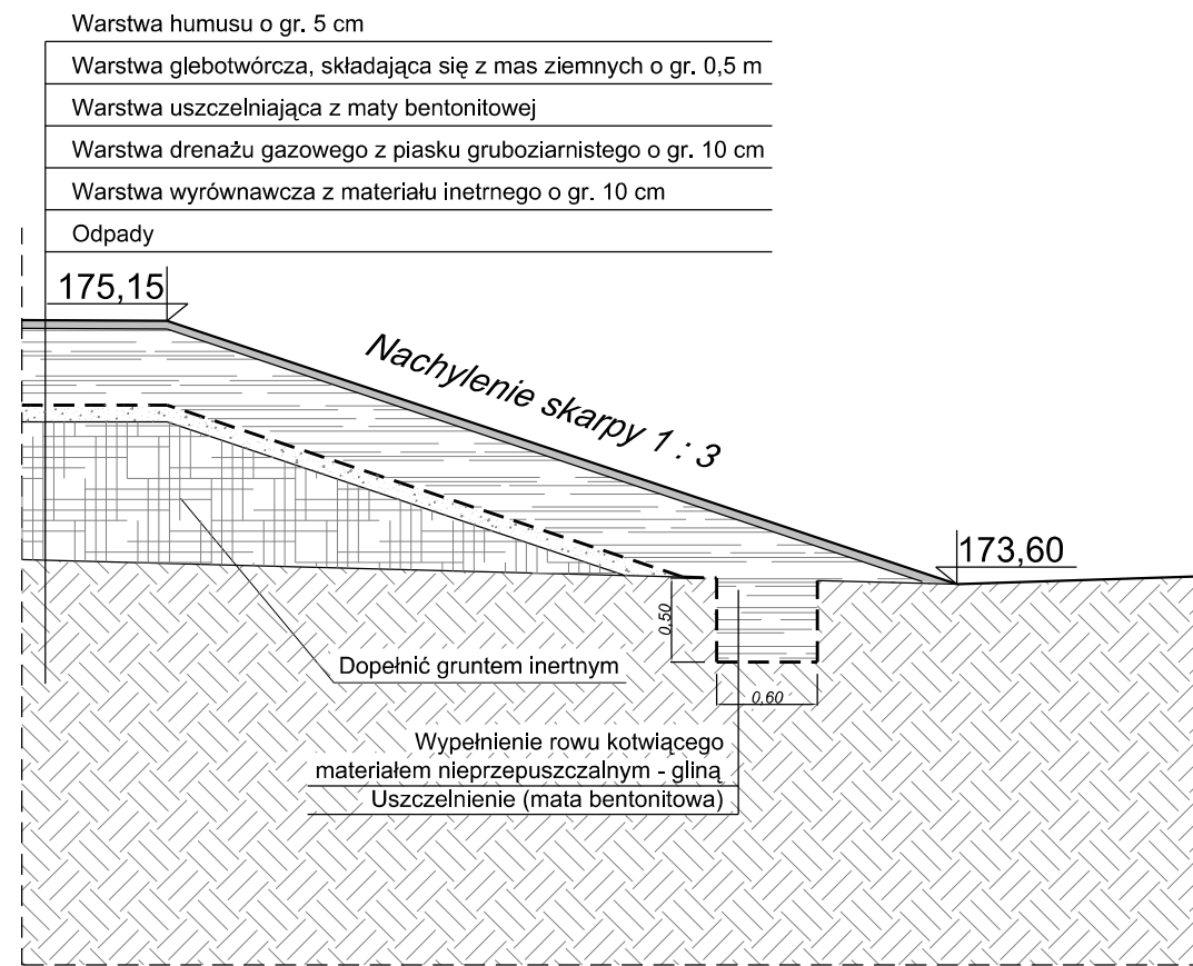
SZCZEGÓŁ "B" 1 : 50
